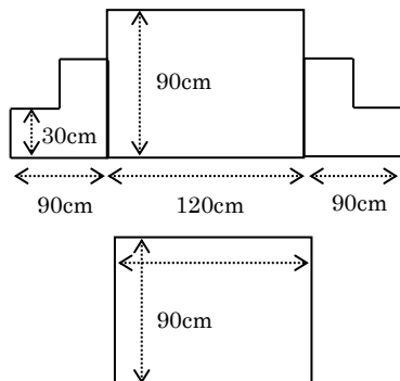
指揮台(大)
